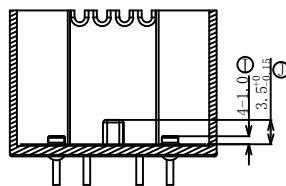
断面 B-B
