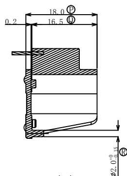
断面 A-A
